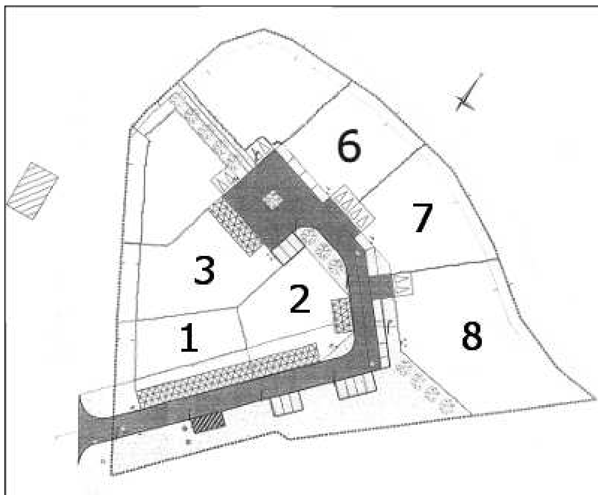
Plan du Lotissement « Hameau du Terberel »
